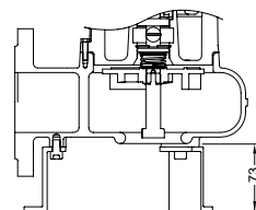
MF 565 с 665 с 3 опорными лапами
